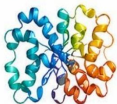
Alpha-Amylase
